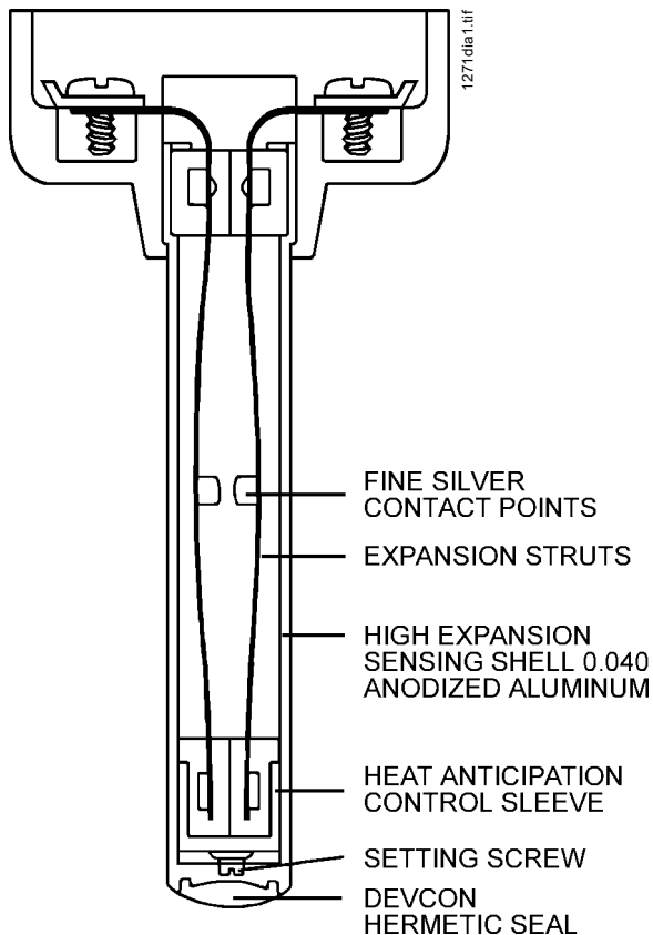
Cut-Away View, ACTUAL SIZE
